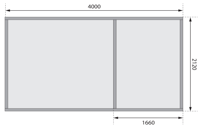
Fundamentplan ohne Boden (in mm)
