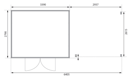
Fundamentplan ohne Boden (in mm)
