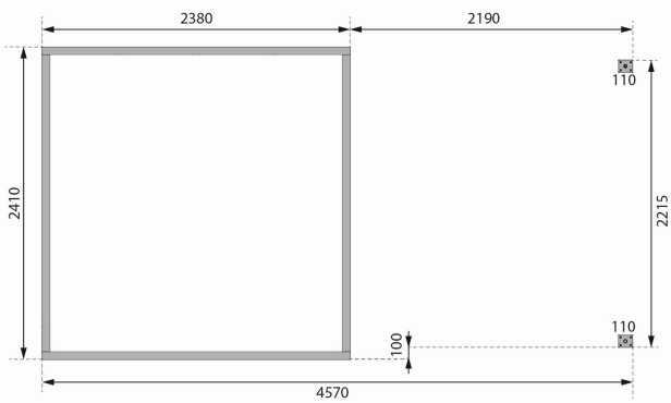
Fundamentplan ohne Boden (in mm)
