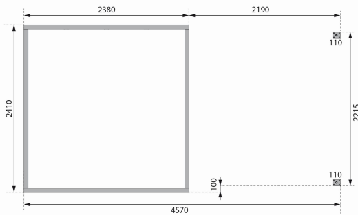
Fundamentplan ohne Boden (in mm)
