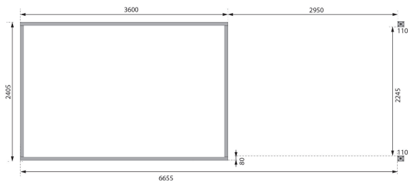
Fundamentplan ohne Boden (in mm)
