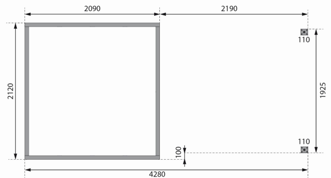
Fundamentplan ohne Boden (in mm)
