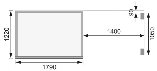
Fundamentplan ohne Boden (in mm)
